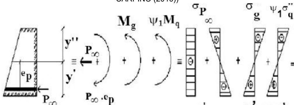
Figura 6 – Verificação ELS-D - Combinação Frequente, Protensão Completa (PEREIRA E CARPINO (2016))
