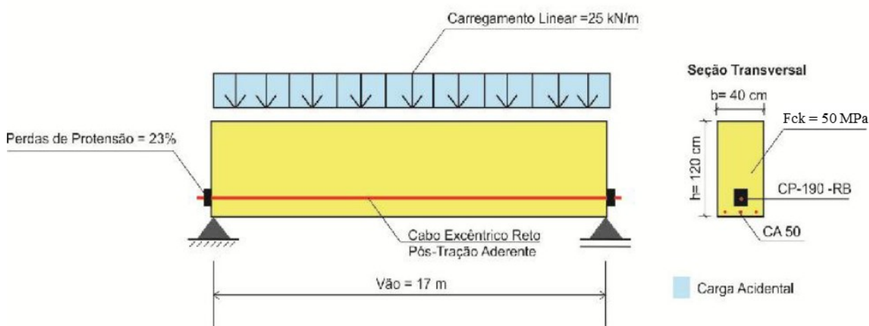
Figura 1 - Viga adotada (Fonte: o autor)
