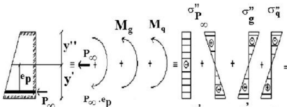
Figura 5 – Verificação ELS-F - Combinação Rara, Protensão Completa (PEREIRA E CARPINO (2016))
