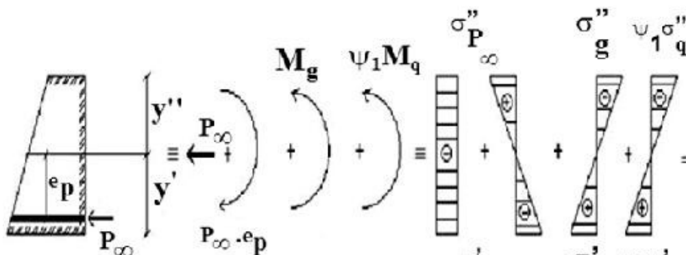
Figura 3 – Verificação ELS-F - Combinação Frequente, Protensão Limitada (PEREIRA E CARPINO (2016))
