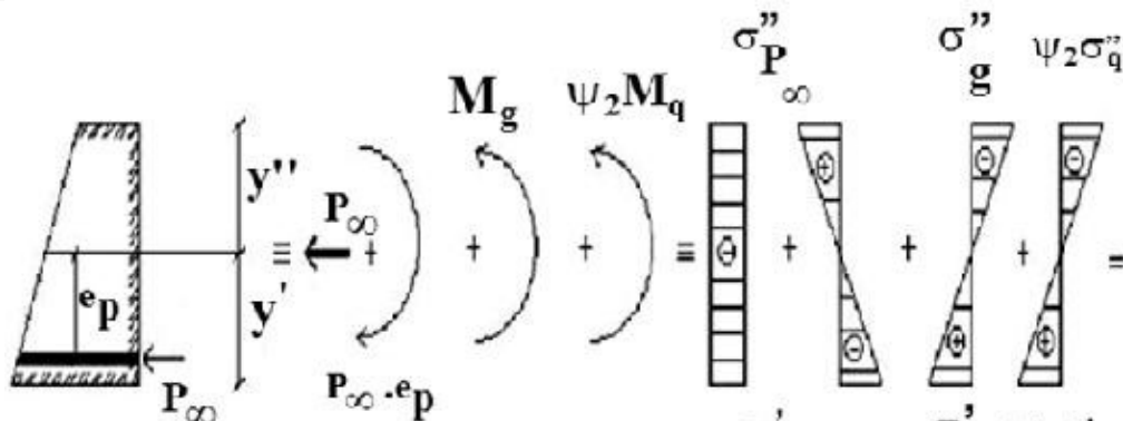
Figura 4 – Verificação ELS-D - Combinação Quase Permanente, Protensão Limitada (PEREIRA E CARPINO (2016))
